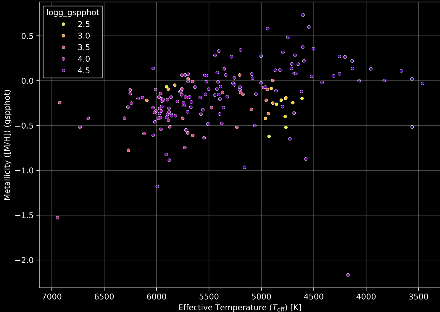
APOGEE DR17 Field: [145+62_MGA] Stellar Population Parameters (n= 181)
